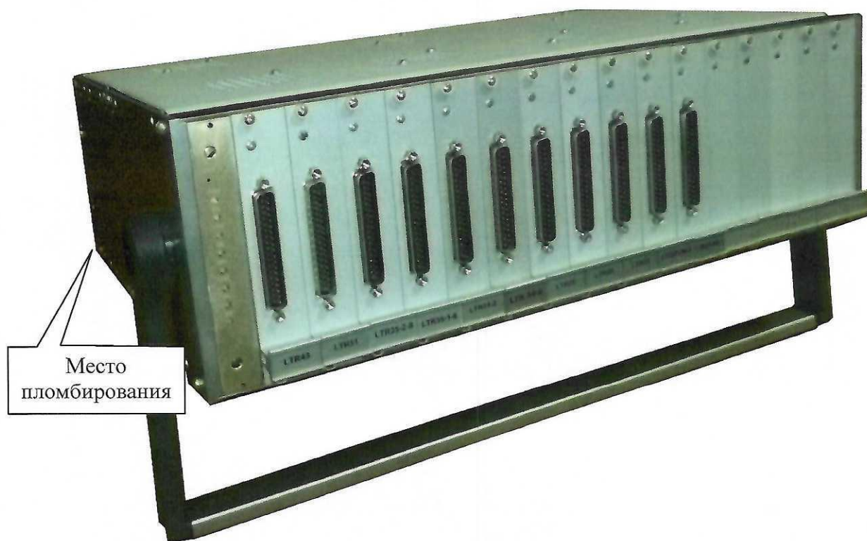
Рисунок 7 – Общий вид установок LTR-AEU-16 и место пломбирования от несанкционированного доступа
