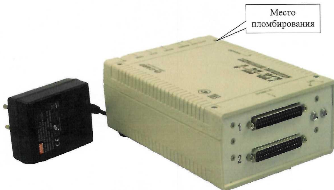
Рисунок 3 – Общий вид установок LTR-EU-2 и место пломбирования от несанкционированного доступа
