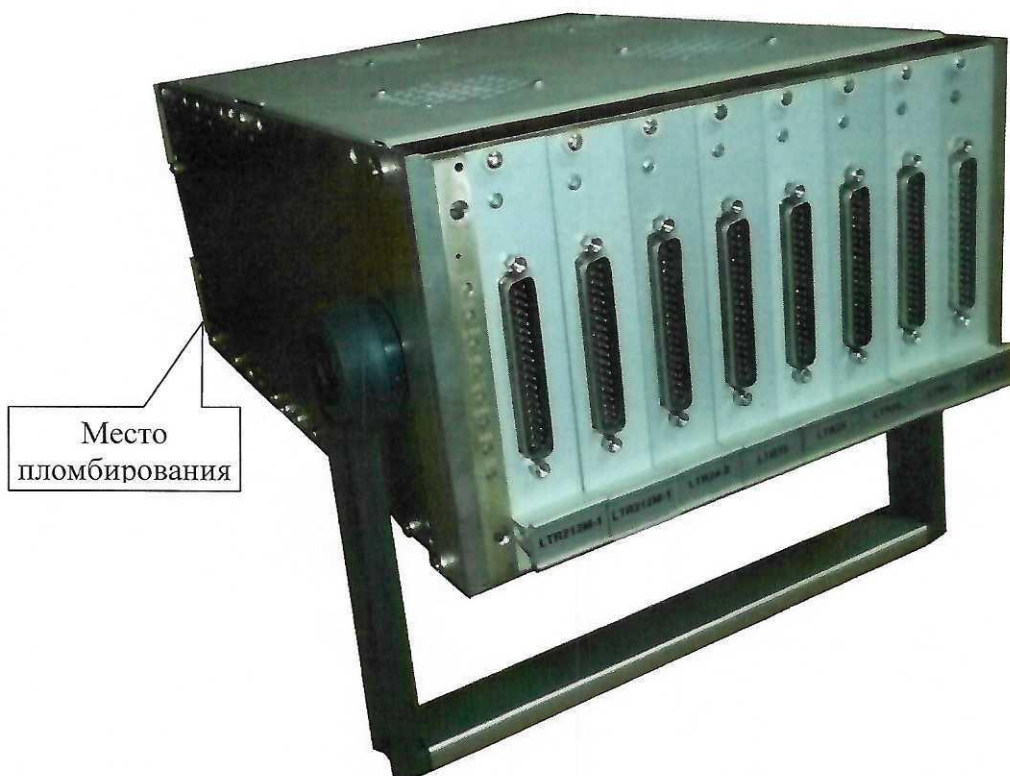
Рисунок 5 – Общий вид установок LTR-BEU-8 и место пломбирования от несанкционированного доступа
